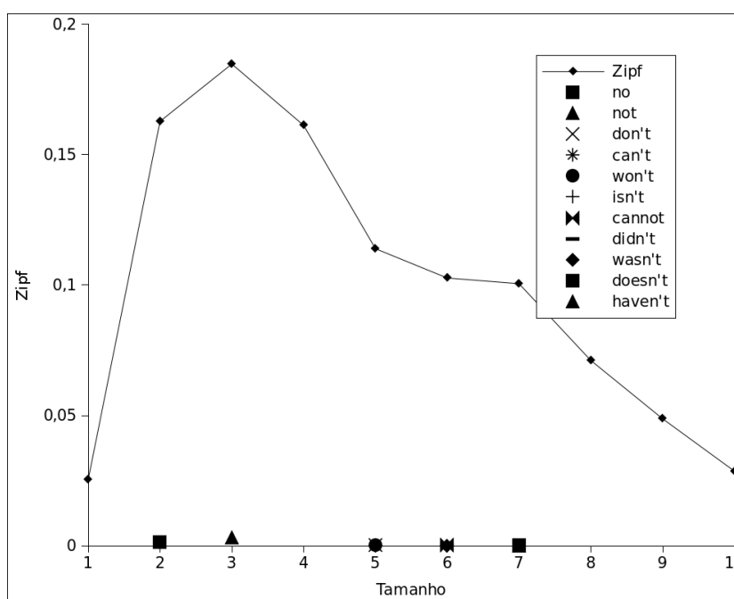
Figura 3.4: Gráfico da frequência relativa para o português
