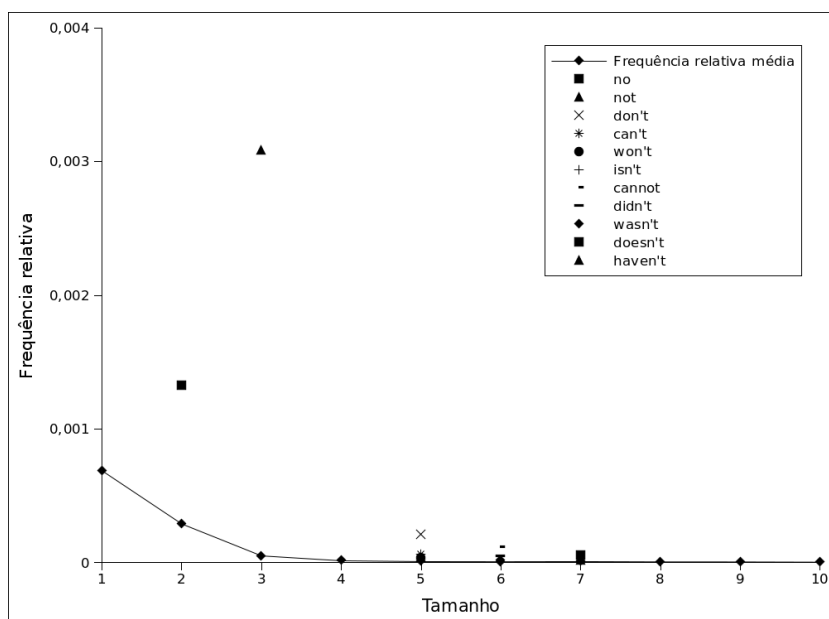
Figura 3.6: Gráfico da frequência relativa para o inglês
