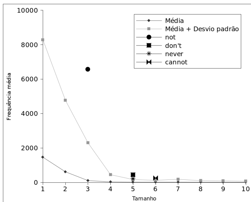
Figura 3.2: Gráfico da frequência média das palavras em inglês
